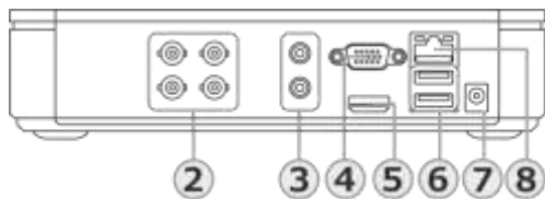
2 Входные разъемы BNC для подключения камер 3 RCA разъемы аудиовход/аудиовыход 4 VGA порт 5 HDMI порт 6 USB 2.0 7 Разъем питания 12 В DC 8 RJ-45 разъем LAN
